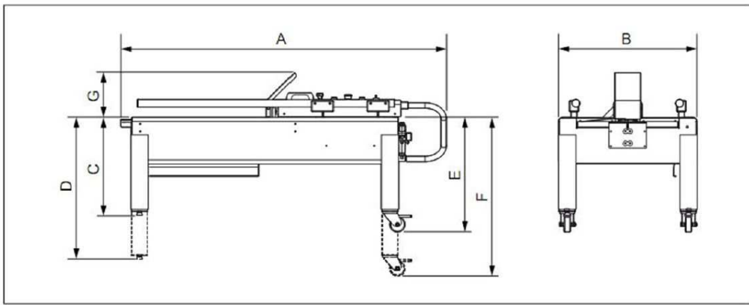
DIMENSIONS et ENCOMBREMENT de la STARBOX 50 et 65
